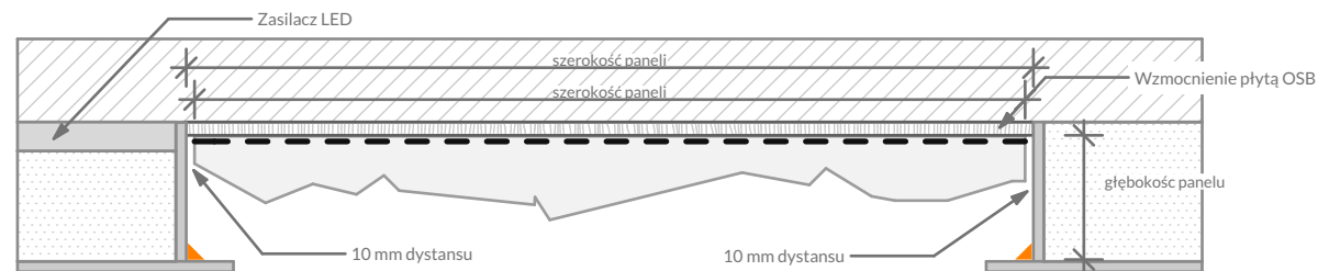
Detal C - widok z góry
