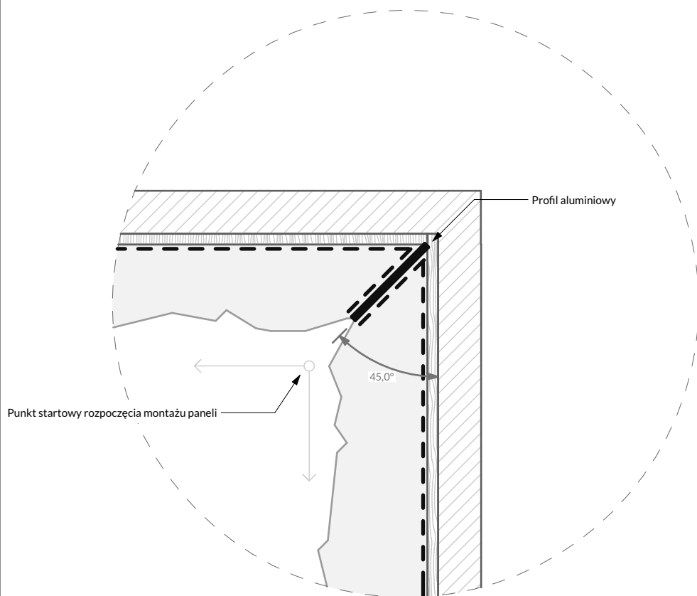
Detal A - narożnik wewnętrzny
