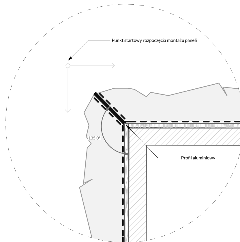
Detal B - narożnik zewnętrzny
